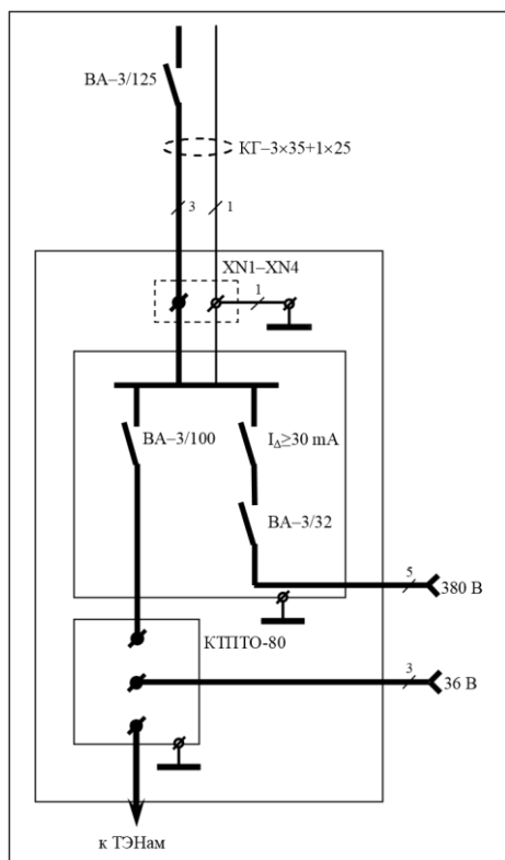
Рисунок 4. Схема электрическая принципиальная дооборудования КТПТО-80.
