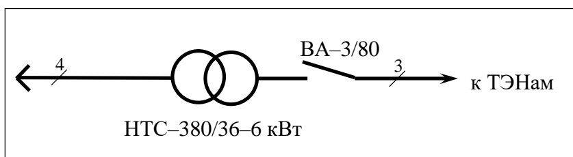
Рисунок 5. Схема электрическая принципиальная дооборудования НТС-380/36-6.0.
